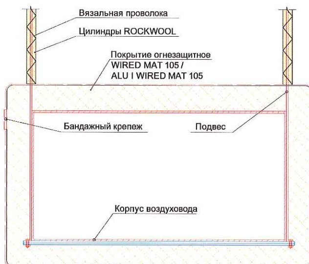
Рис. 9. Принципиальная схема изоляции подвесов.
