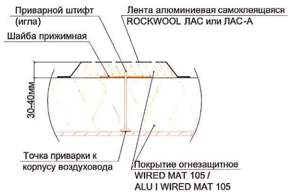
Узел 1.1
