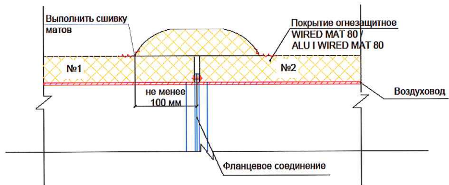
Рис. 6. Установка изоляции на фланец укрупненного блока воздуховода
