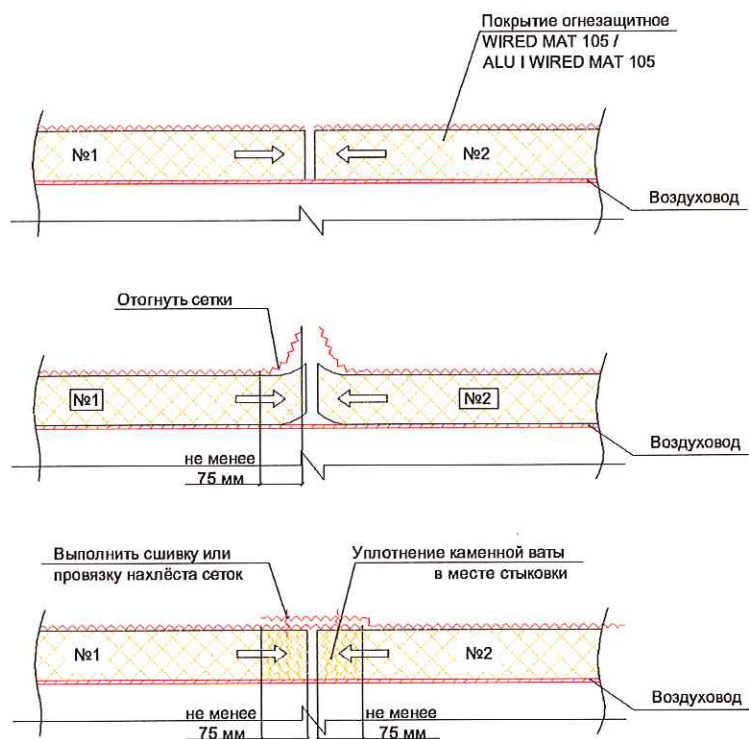
Рис. 5.1. Выполнение припуска с последующим уплотнением.
