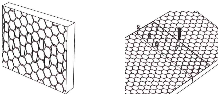
Рис. 3 Использование вязальной проволоки и вязального крючка для крепления матов WIRED MAT
