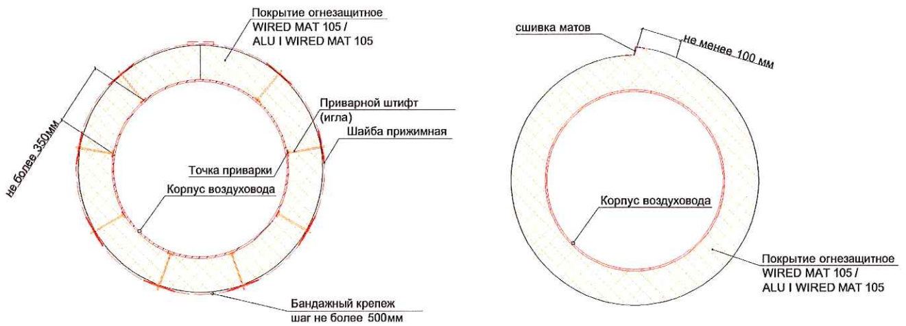
Узел 1.1
