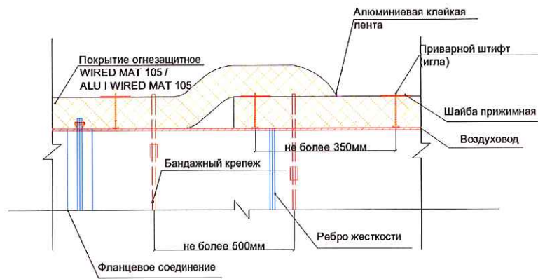
Рис. 5. Выполнение нахлеста не менее 150 мм материала огнезащитного покрытия.
