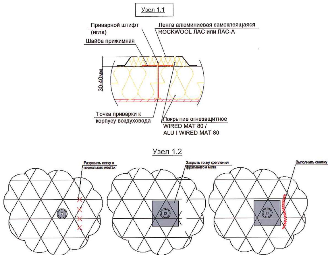
Рис. 4. Принципиальная схема расположения матов по периметру воздуховода прямоугольного и круглого сечения
