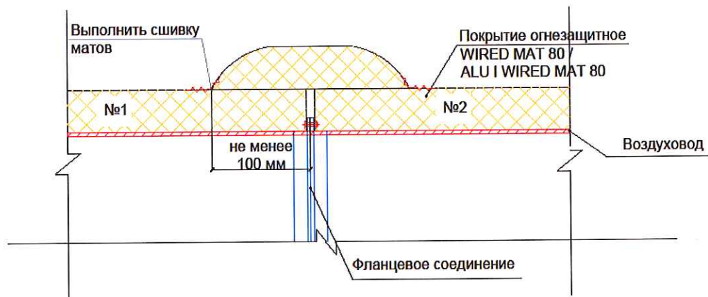
Рис. 6. Установка изоляции на фланец укрупненного блока воздуховода
