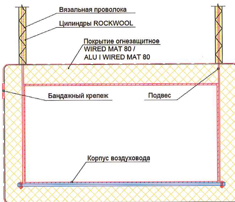
Рис. 8. Принципиальная схема изоляции подвесов.
