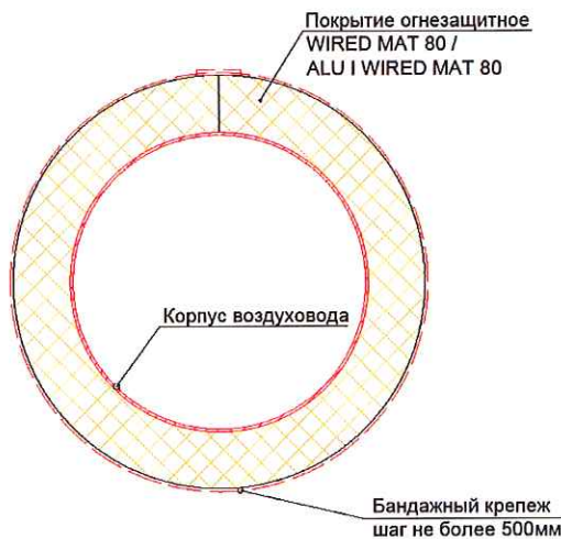
Рис. 7 а, б. Крепление огнезащитного покрытия WIRED MAT 80 / ALU I WIRED MAT 80 к воздуховоду с помощью бандажного крепежа или вязальной проволоки диаметром 2,0 – 3,0 мм.
