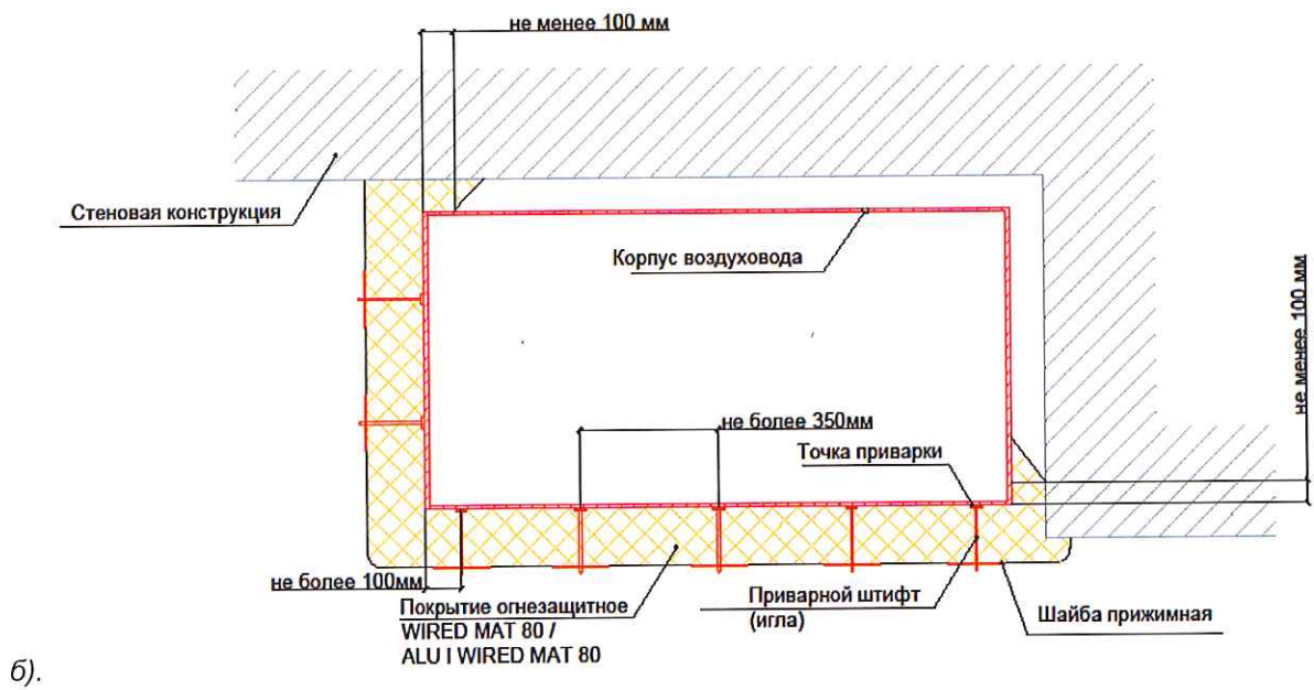
Рис. 6 а, б Огнезащита воздуховода, расположенного вблизи стеновых конструкций
