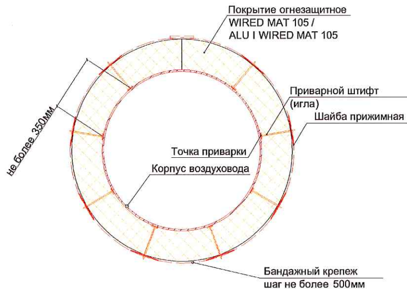
Рис. 8 а и б. Крепление огнезащитного покрытия комбинированным способом.
